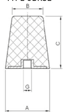
TYPE GBKSE
